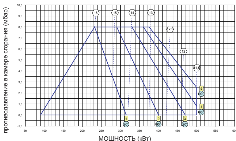
ПРИМЕР ПРЕДВАРИТЕЛЬНОЙ КАЛИБРОВКИ JOB 50/2
