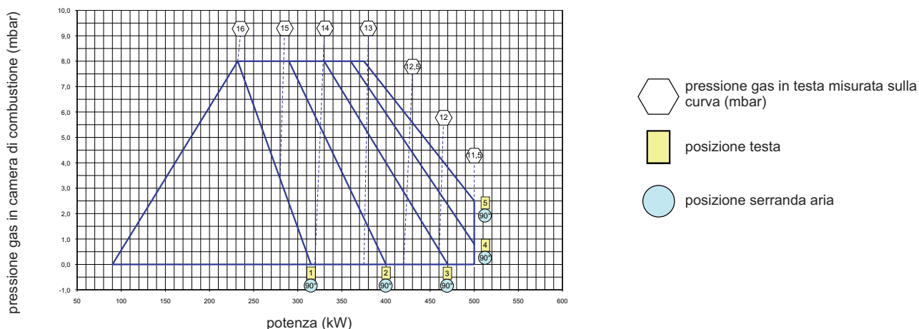
ESEMPIO DI PRETARATURA JOB 50/2
