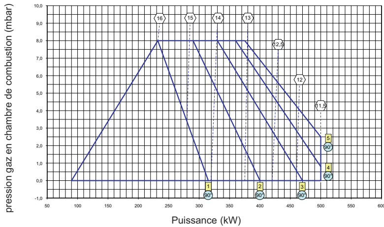
EXEMPLE DE PREREGLAGE JOB 50/2
