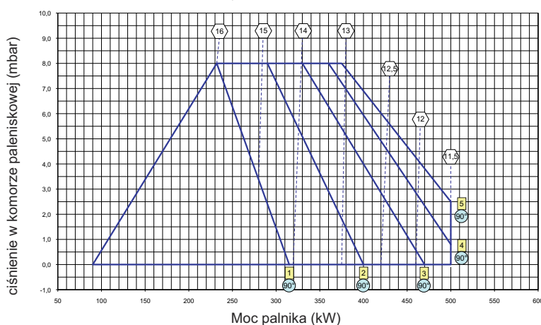
PRZYKŁAD WSTĘPNEJ KALIBRACJI JOB 50/2
